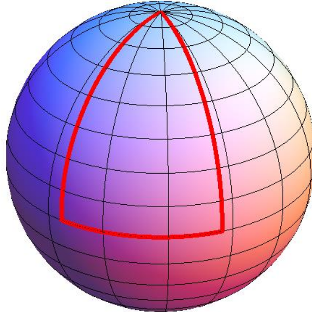
Sphärische Geometrie
