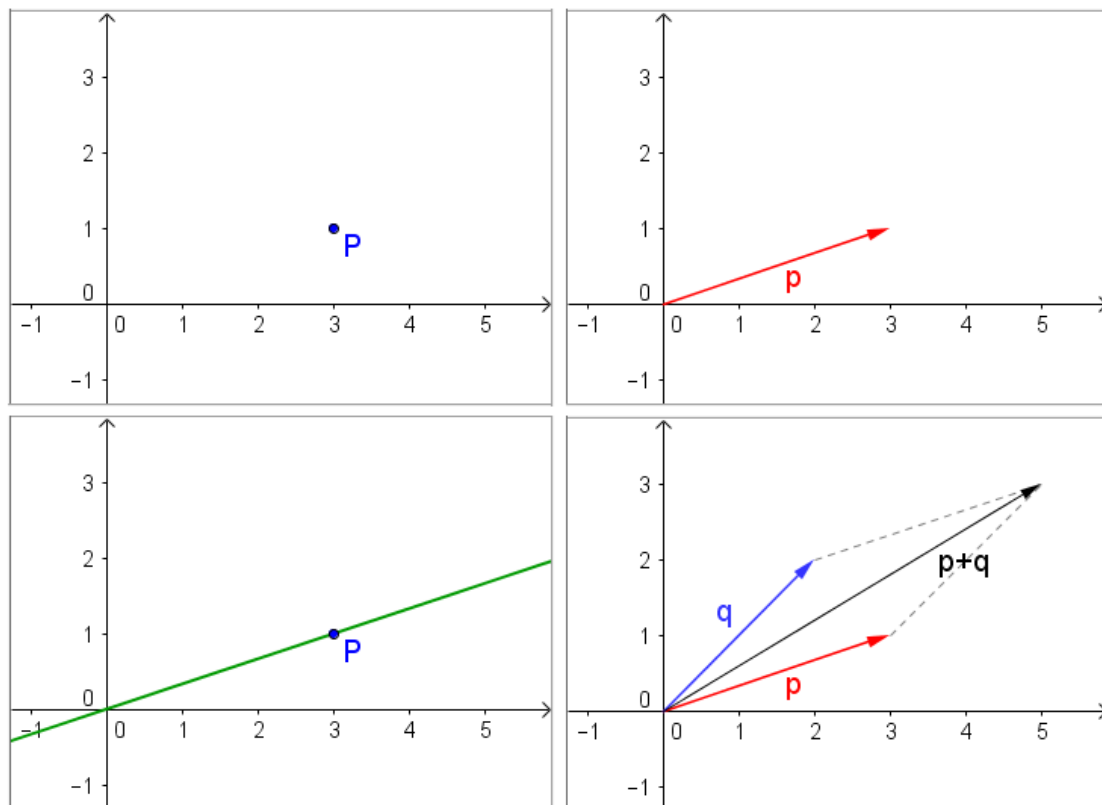
Abbildung 1: Die Deutung reeller Zahlenpaare als Punkte – links oben das Zahlenpaar (3, 1) gedeutet als Punkt – ist nützlich etwa zur Charakterisierung von Teilmengen des \mathbb{R}^2 . So stellt beispielsweise die grüne Gerade (links unten) die Menge aller Vielfachen von (3, 1) dar. Die Deutung reeller Zahlenpaare als Pfeile – rechts oben das Zahlenpaar (3, 1) gedeutet als Pfeil – ist nützlich zur Visualisierung der Vektorraum-Operationen. Als Beispiel ist rechts unten die Visualisierung der Addition (3, 1) + (2, 2) = (5, 3) dargestellt.
