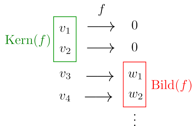
Abbildung 2: Schematische Skizze des soeben bewiesenen Sachverhalts. Die Punkte deuten an, dass der Zielvektorraum W Elemente enthalten kann, die nicht von f getroffen werden. Die Dimension von W muss mindestens 2 sein, kann aber durchaus größer sein.
