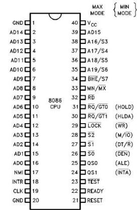
Abbildung 3: Pinbelegung 8086 (Quelle: https://commons.wikimedia.org/w/index.php?curid=7895244
