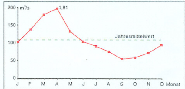
Abb. 5: Jahresganglinie Abflussmenge, Pegel Angern (1951-1980). 1,81: Verhältnis von Monatsmittelwert des abfließendsten Monats zu Jahresmittelwert (nach ZULKA 1991, aus HÖDL & RIEDER 1993a).
